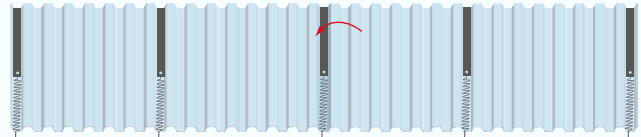
Bevestiging met bevestigingsband voor kap n° 5 en groter
