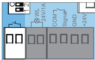
Afb. Aansluiting drukknop
